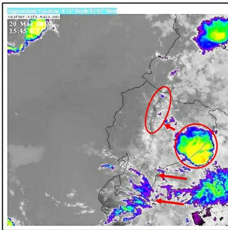
Imagen Satelital IR del GOES-16 / 20 de marzo / 10:45 am
